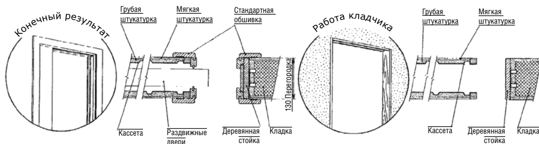
Рис 2.1 Перегородка 125мм — стандартная обшивка
