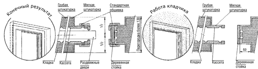
Рис 2.3 Кладка более 125мм — стандартная обшивка Симметричное встраивание кассеты
