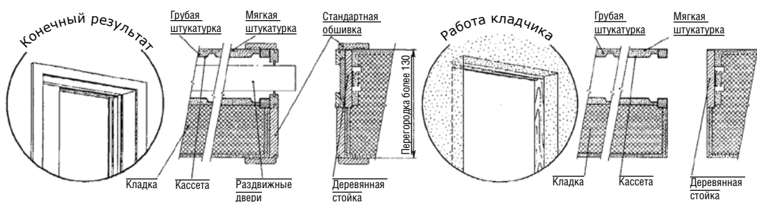
Рис 2.4 Кладка более 125мм — нестандартная обшивка Асимметричное встраивание кассеты
